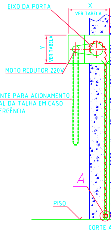
CORTE AA
